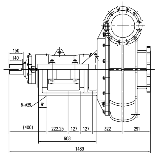
Discharge Flange
