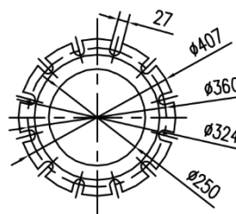
Discharge Flange
